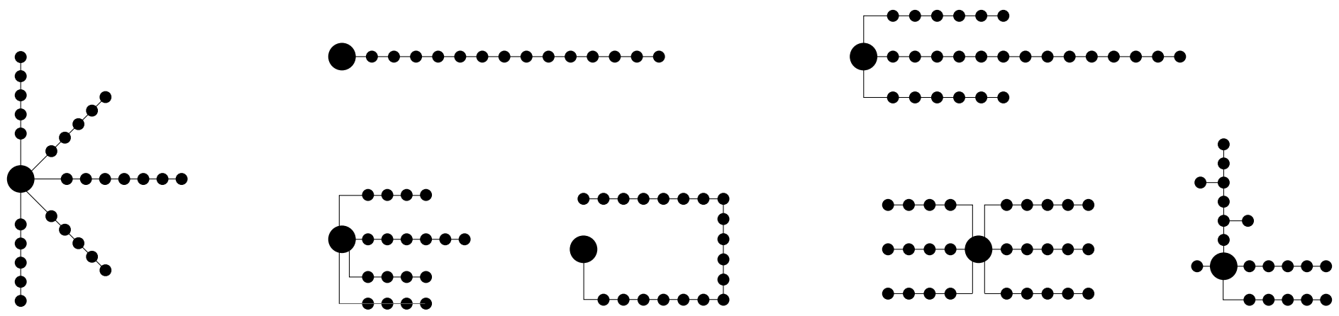
Przykładowe topologie magistrali TUKAN [Łączna długość przewodu max. 400m]
