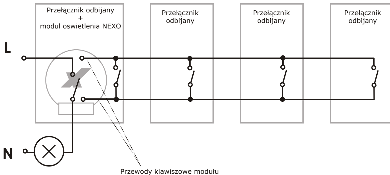
Łączniki świecznikowe odbijane
