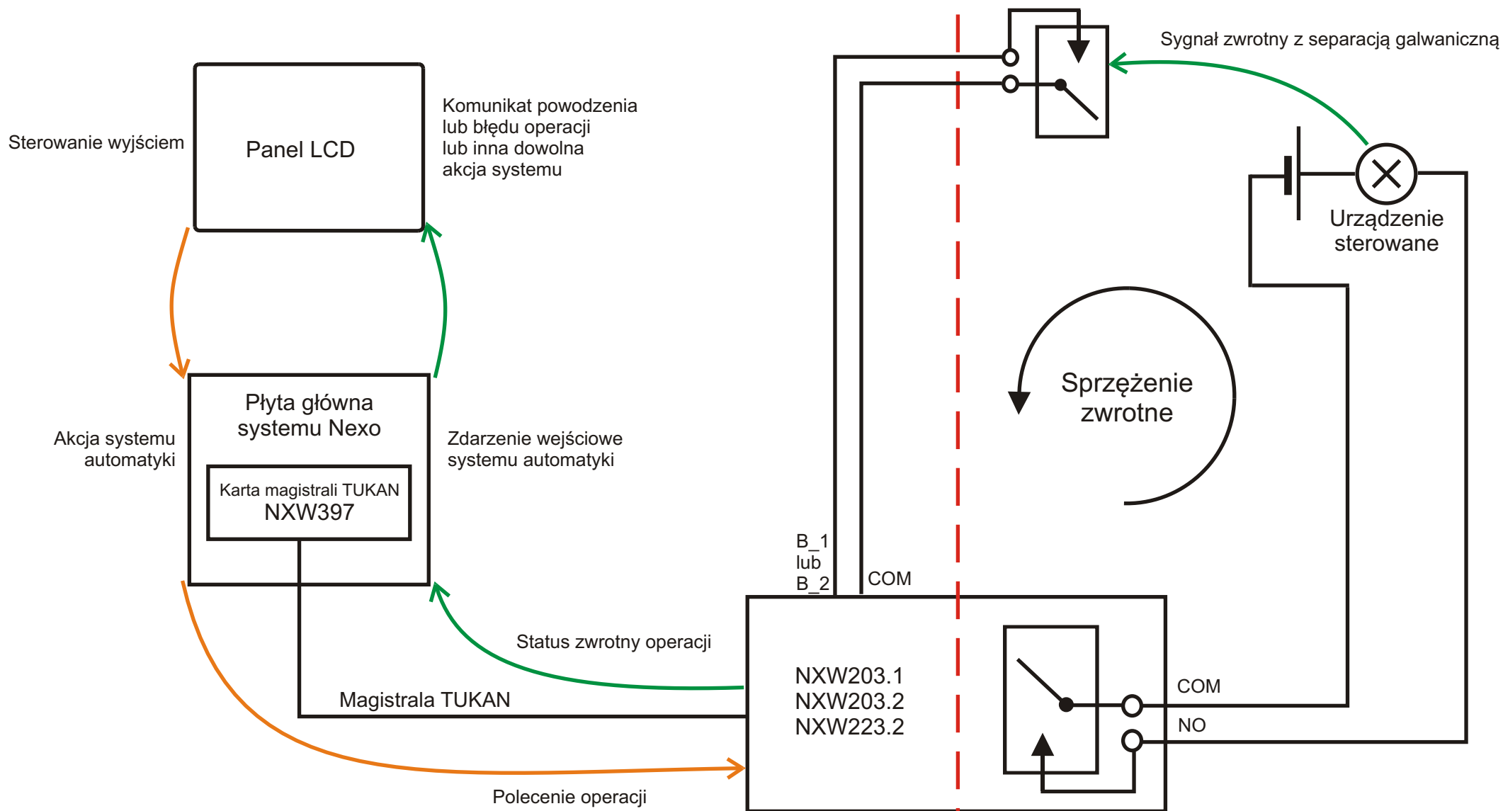
Pojedynczy obwód przekaźnika z funkcją potwierdzenia załączenia obwodu
